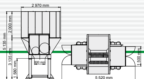
Concasseur double arbres de type 489 Quebradora de dos ejes Tipo 489
