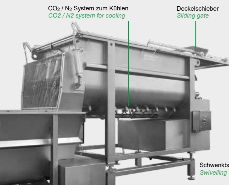
▼ KS Mischer 2000 Typ 750 KS Mixer 2000 Type 750
