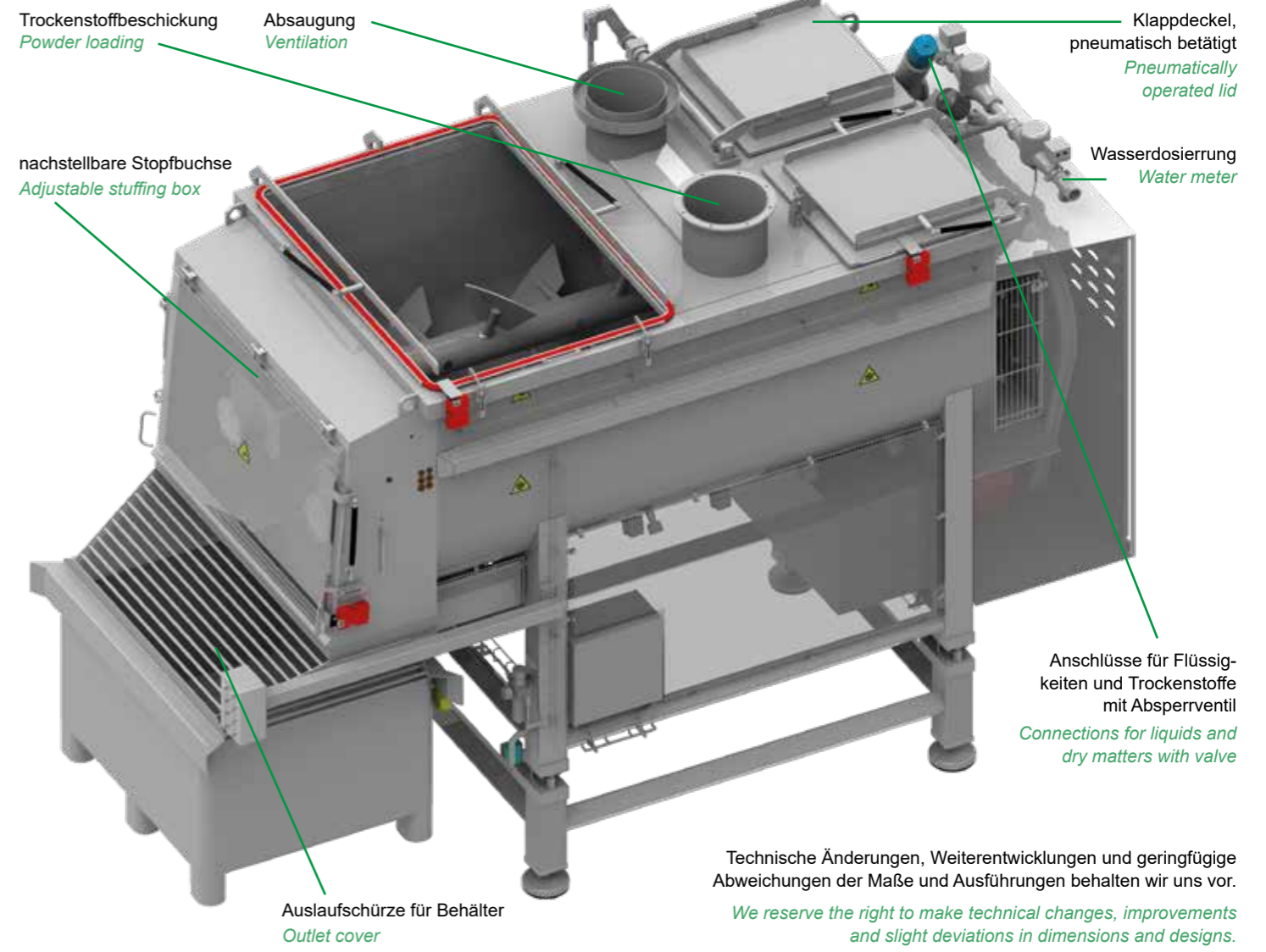
▼ KS Mischer 400 Typ 770 KS Mixer 400 Type 770
