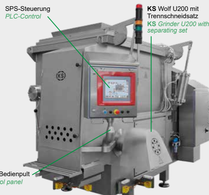
▼ KS Mischwolf 1000 Typ 751 KS Mixer Grinder 1000 Type 751
