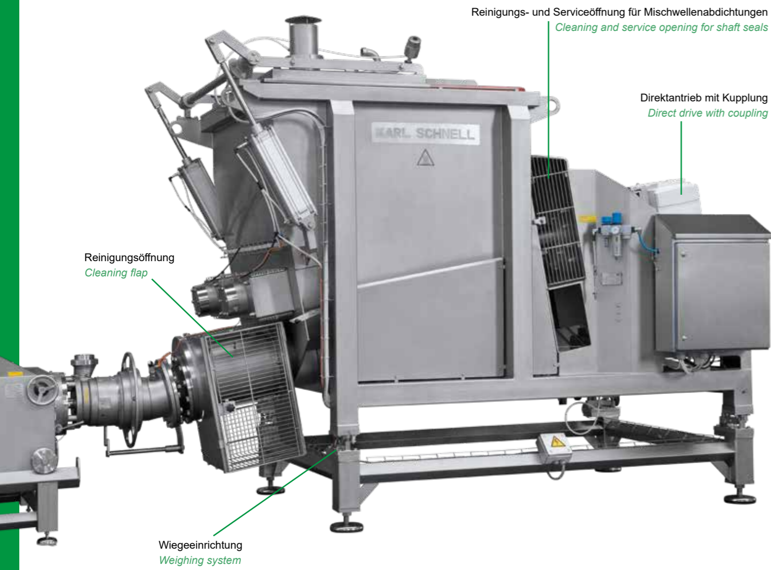
▼ KS Mischer 2000 Typ 750 KS Mixer 2000 Type 750
