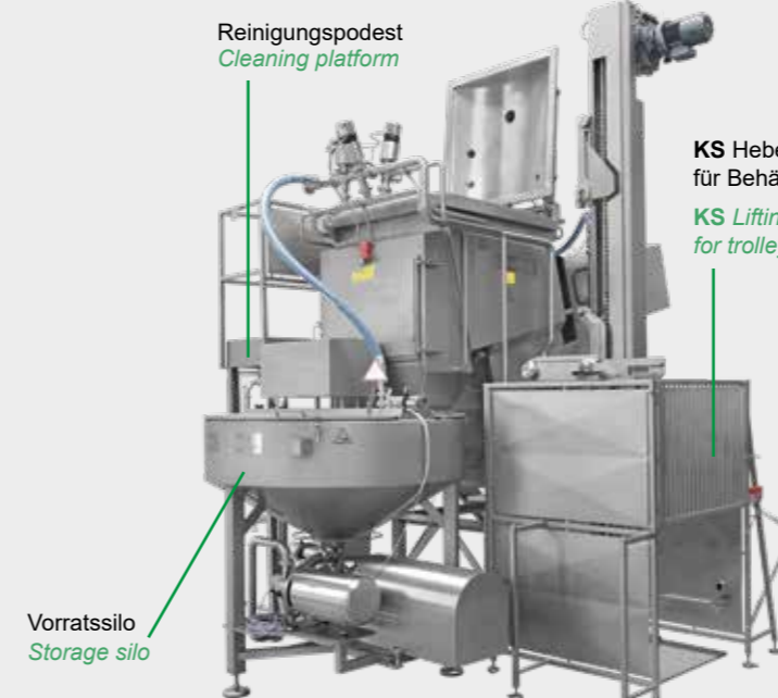
▼ KS Mischer 400 Typ 770 KS Mixer 400 Type 770
