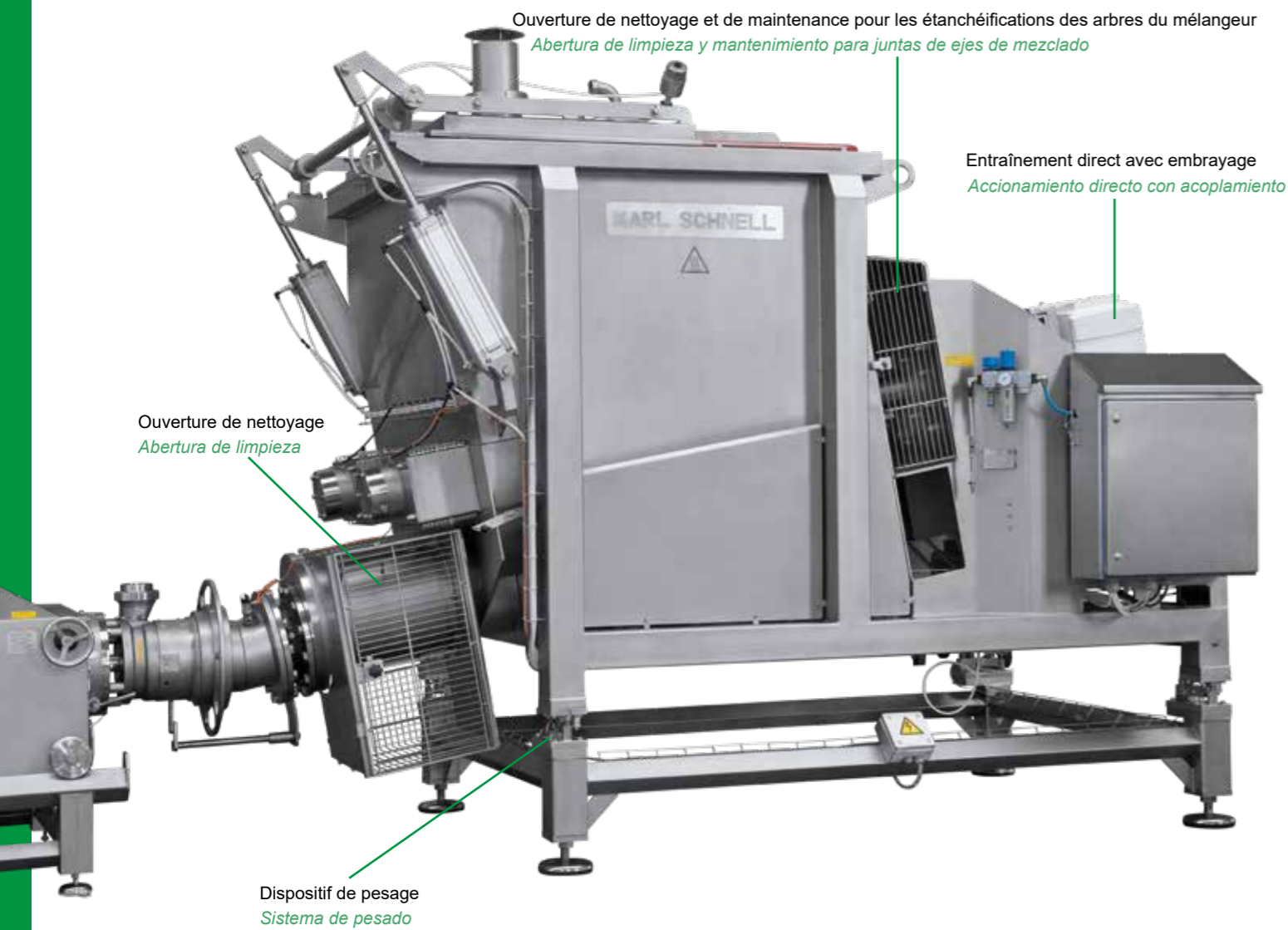
▼ Mélangeur KS 2000 Type 750 Mezcladora KS 2000 Tipo 750
