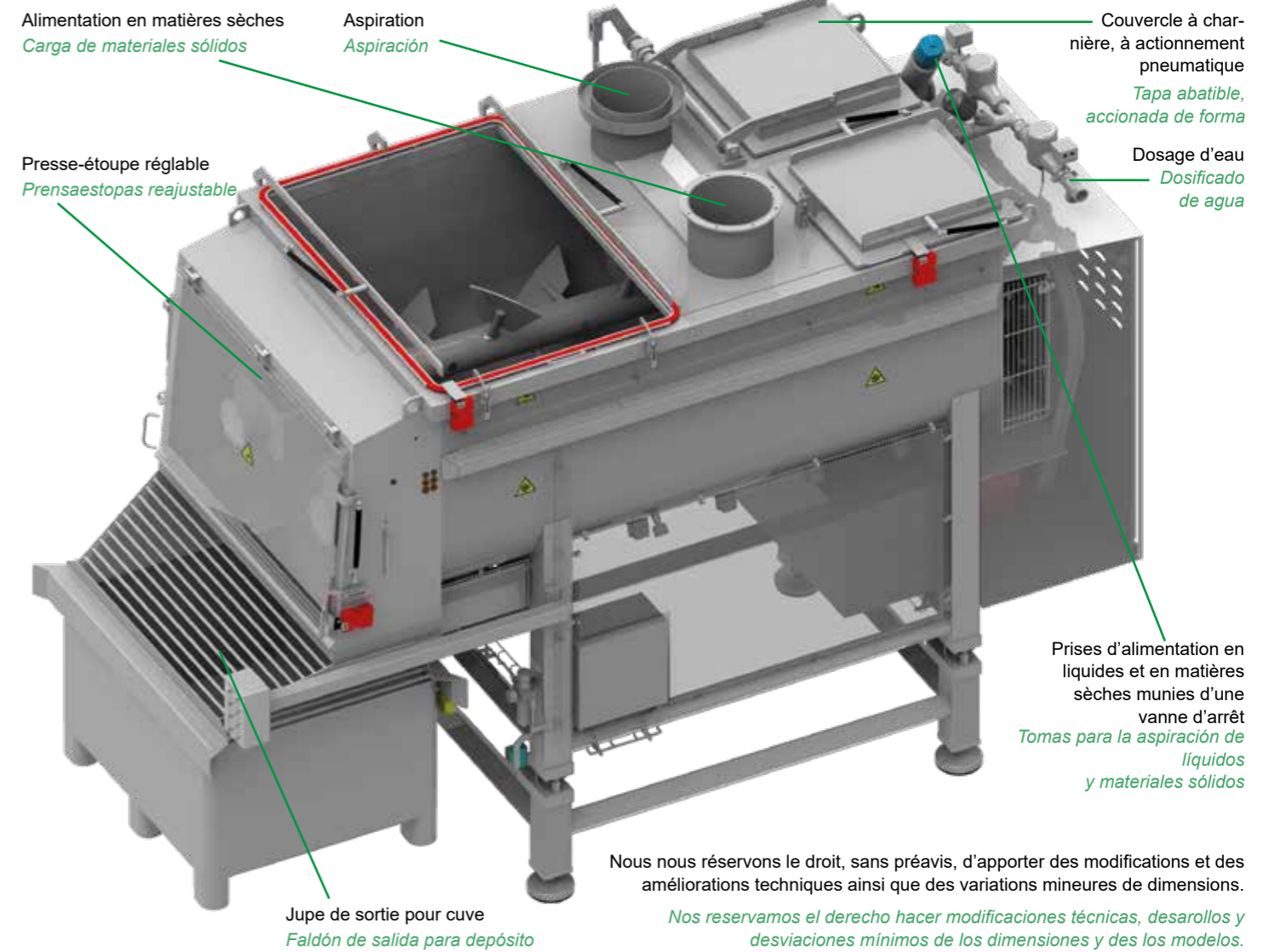
▼ Mélangeur KS 400 Type 770 Mezcladora KS 400 Tipo 770
