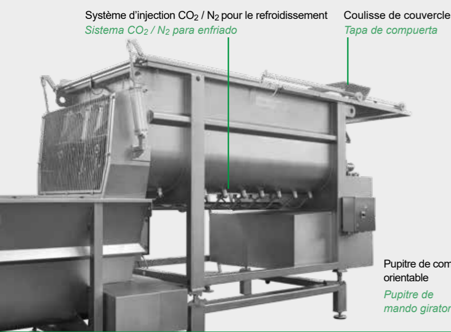
▼ Mélangeur KS 2000 Type 750 Mezcladora KS 2000 Tipo 750
