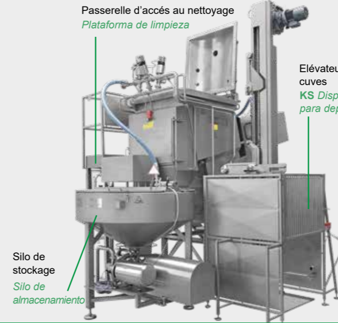
▼ Mélangeur KS 400 Type 770 Mezcladora KS 400 Tipo 770
