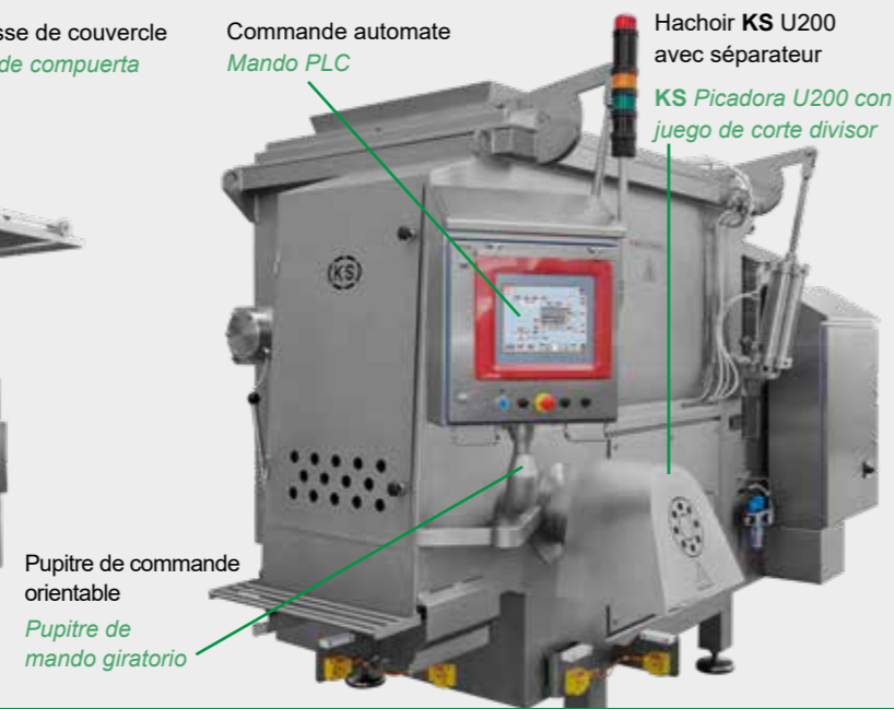
▼ Mélangeur-broyeur KS 1000 Type 751 Mezcladora KS 1000 Tipo 751
