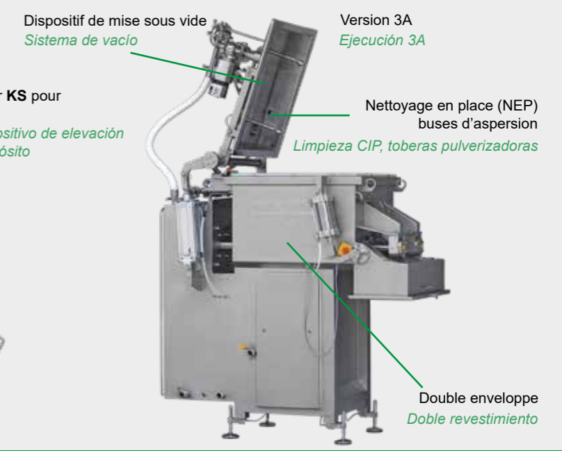
▼ Mélangeur KS 200 Type 770 Mezcladora KS 200 Tipo 770
